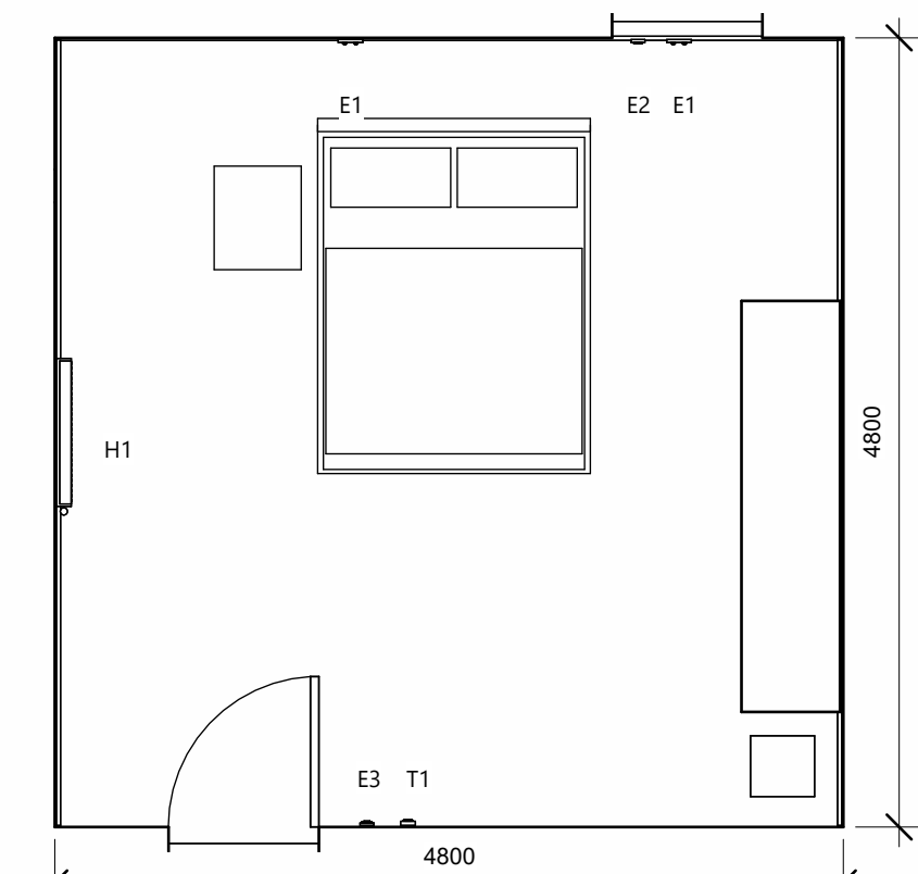
1 A-203_RD FP 1 : 50
