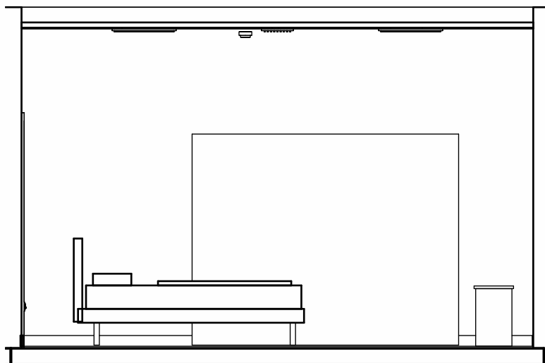
6 A-203_RD E_03 1 : 50
